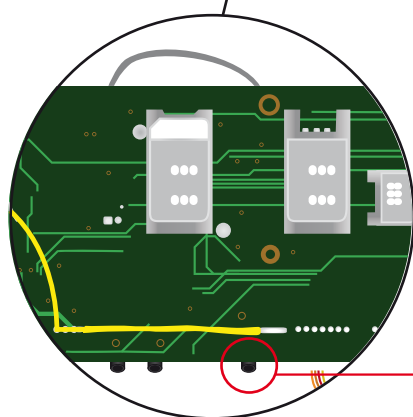
Vista trasera placa U+PRO
