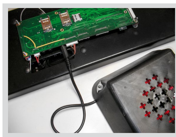
Plug ficha conectada a la placa U+PRO
